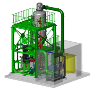
MVR 蒸留濃縮装置
