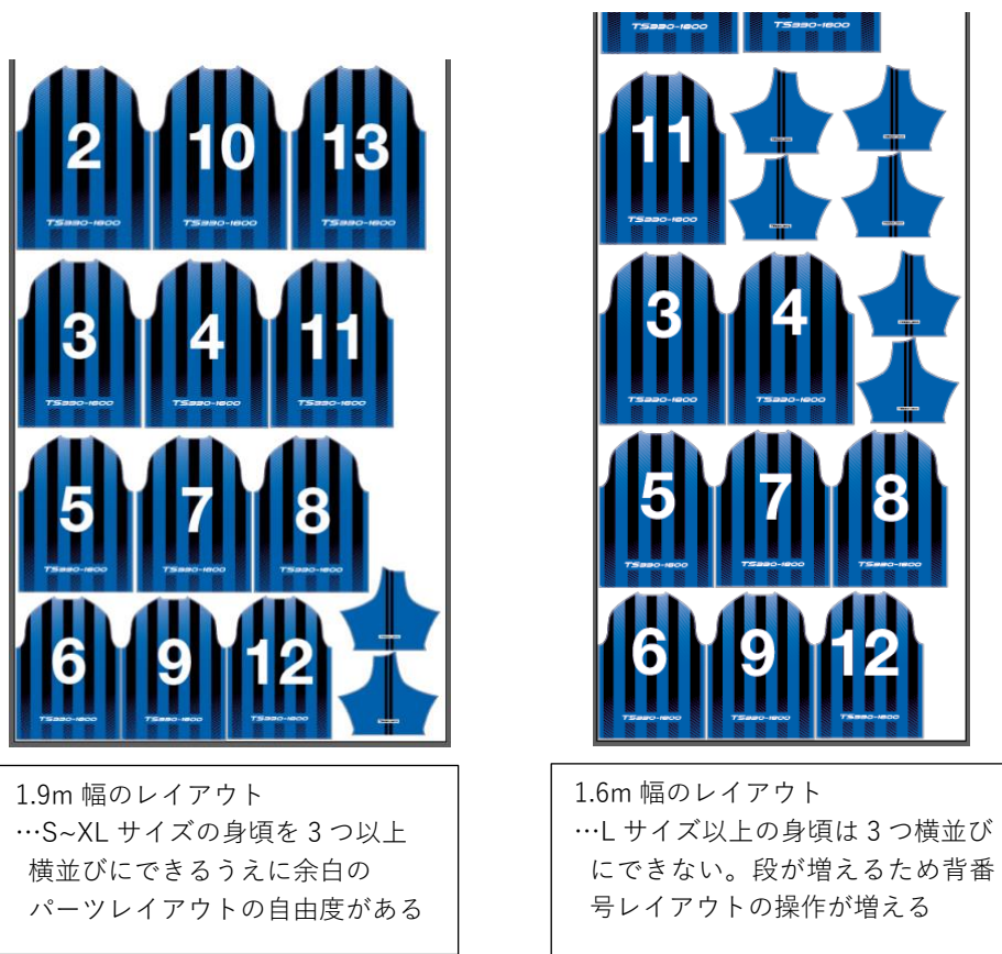
図1 スポーツユニフォームの型紙配置のイメージ ※S~XL サイズを各 3 着制作する場合
