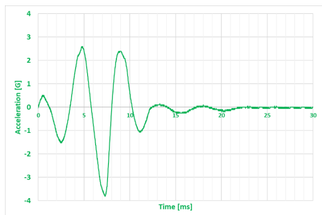
振動波形例
