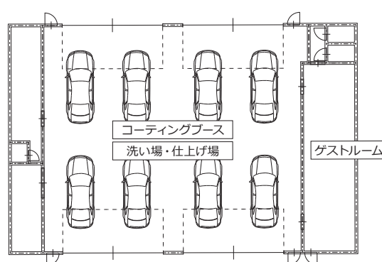
【店舗平面図】
