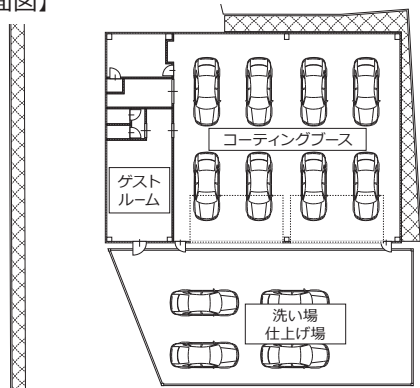
【店舗平面図】
