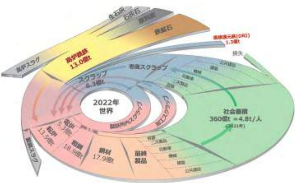
〔鉄の資源循環(クローズドルプリサイクル)〕
