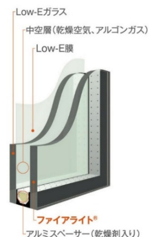
ファイアライトを用いた Low-E 複層ガラスの 構成イメージ
