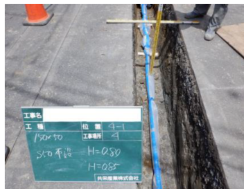
【水道管布設工事】
