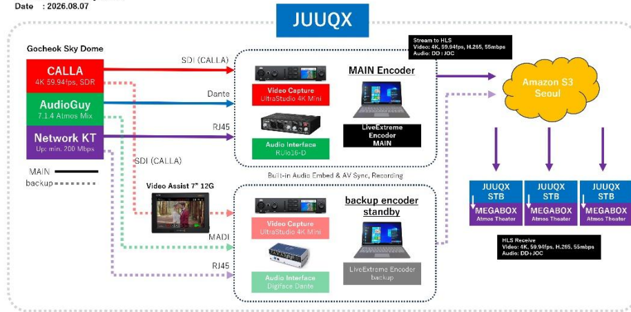
本ライブビューイングの JUUQX システム図
