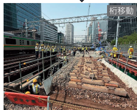
田町駅線路切換工事 (2025/4/19~20)
